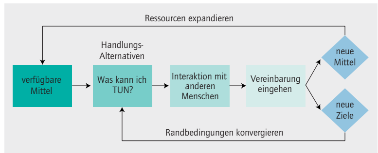
Abb. 1 Effectuation-Prozess unternehmerischen Handelns 7
