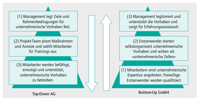
Abb. 3 Vergleich der beiden Vorgehensmodelle
